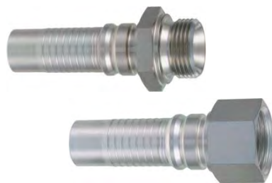
DKR BSP-Gewinde, 60°-Konus BSP thread, 60° cone Seite / page 61
