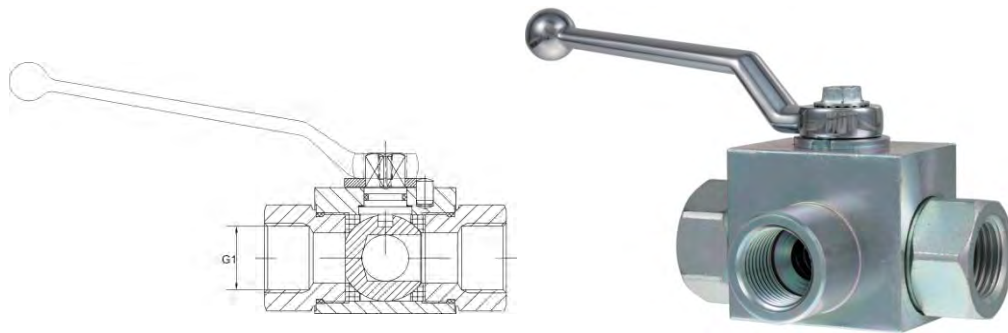
Dreiwegehahn Typ DKH...R / Three way ball valves Type DKH...R BSP-Innengewinde, L- oder T- Bohrung. With female thread BSP.
