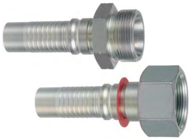
ORFS UNF-Gewinde, flachdichtend UNF thread, flat sealing Seite / page 63
