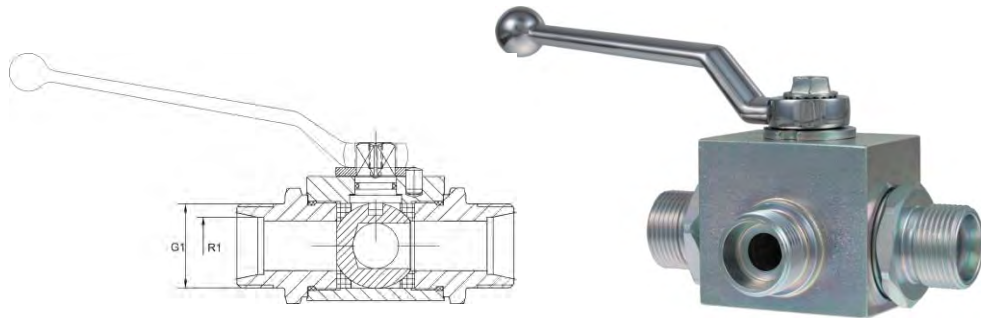
Dreiwegehahn Typ DKH / Three way ball valve Type DKH Metrisches Außengewinde mit 24°-Innenkonus. Male thread 24°.
